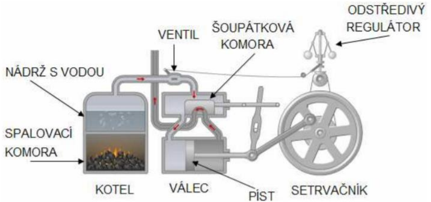
Obr. 3-1 schéma parního stroje [10]
